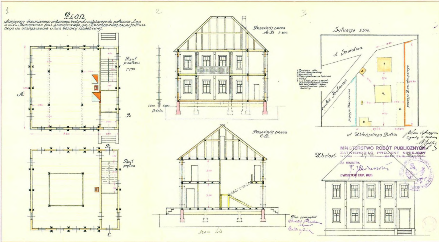
План існуючага драўлянага двухпавярховага будынка спадара Арона Ліса ў мястэчку Ганцавічы Лунінецкага павета Круговіцкай гміны, прызначаны для размяшчэння ізраільскай синагогі, 1926. Друкуецца ўпершыню. Крыніца: Archiwum Akt Nowych. — Zespół "Ministerstwo Spraw Wewnętrznych w Warszawie". Sygnatura 2/9/0/5.5/1 2595.
